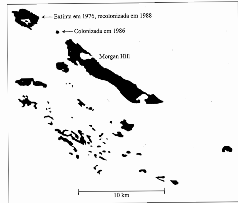
Figura 4.3 Distribuição de prados em solos serpentinos no Condado de Santa Clara, Califórnia. Estas manchas de habitat funcionam como potenciais lugares de populações da borboleta-de-São-Francisco ( Euphydryas editha bayensis ). A grande população de borboletas na localidade de Morgan Hill provavelmente serve como um reservatório contínuo de colonizadores para outras manchas menores, tal como no modelo de ilha-continente. (Baseado em Harrison et al. 1988.)
