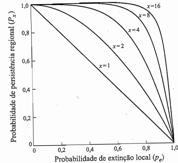
Figura 4.1 Relação entre a probabilidade de persistência regional ( P_x ), a probabilidade de extinção local ( p_e ) e o número de populações ( x ). Note que, à medida que o número de populações aumenta, a probabilidade de persistência regional se torna substancialmente mais alta, para uma determinada probabilidade de extinção local.
